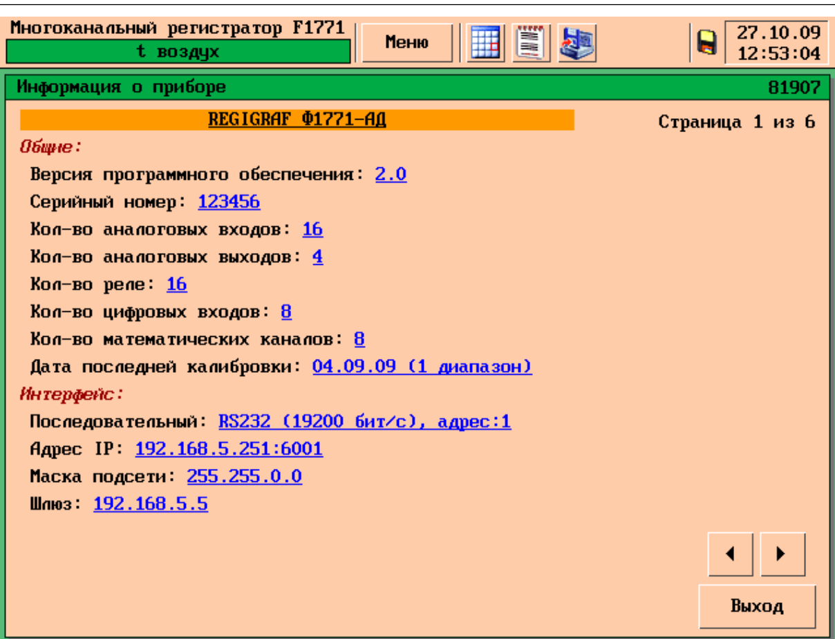
Рисунок 5 – Информация о приборе страница 1: общие настройки прибора и настройки интерфейса
