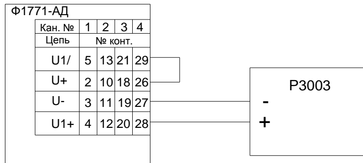
Рисунок 62 - Схема подключения входных каналов для U в диапазонах \pm 10 В
