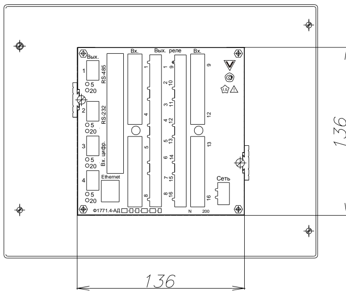
Рисунок 1 – Габаритный чертёж прибора и вырез в щите
