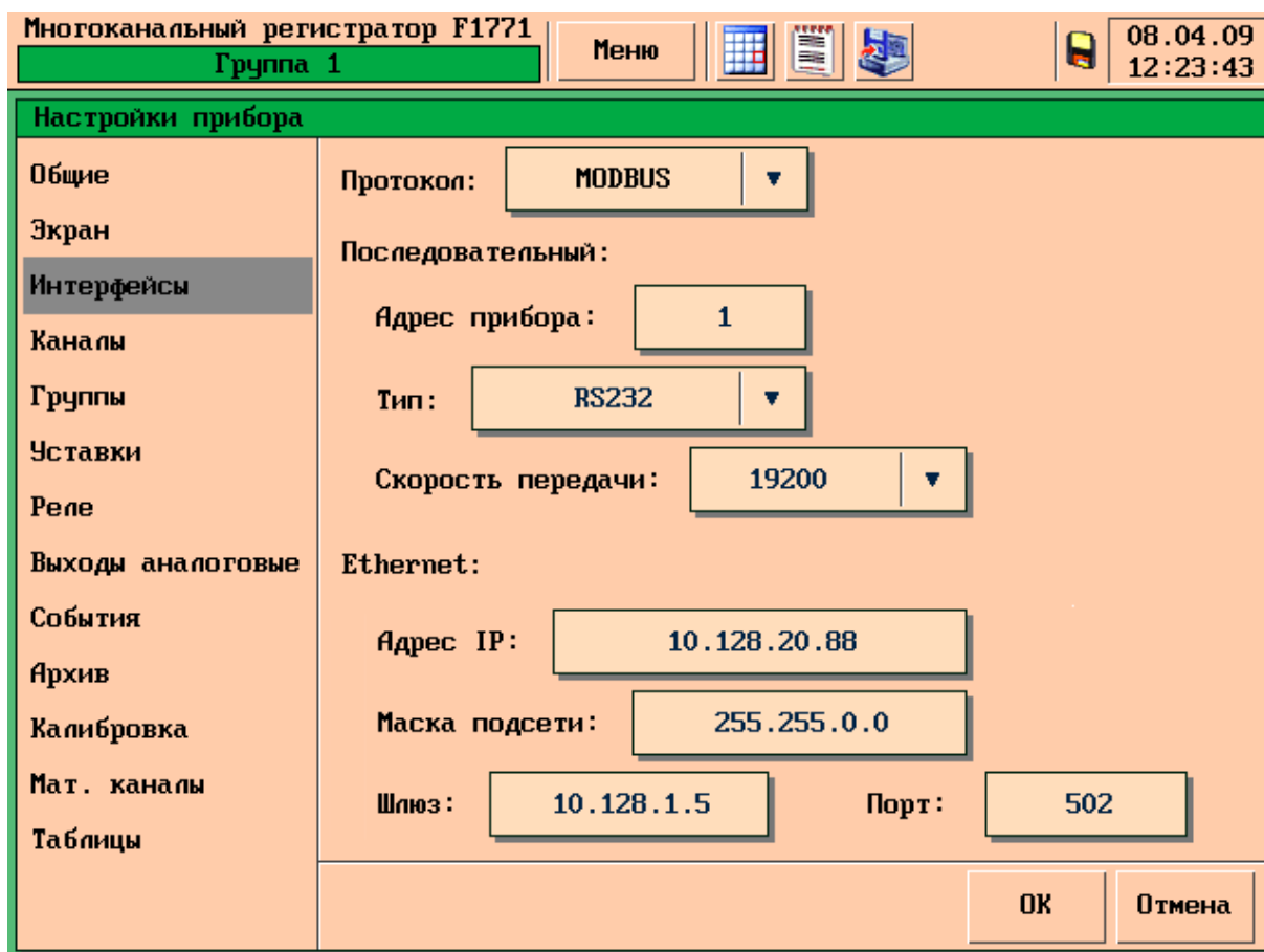
Рисунок 29 – Раздел меню «Интерфейс»
