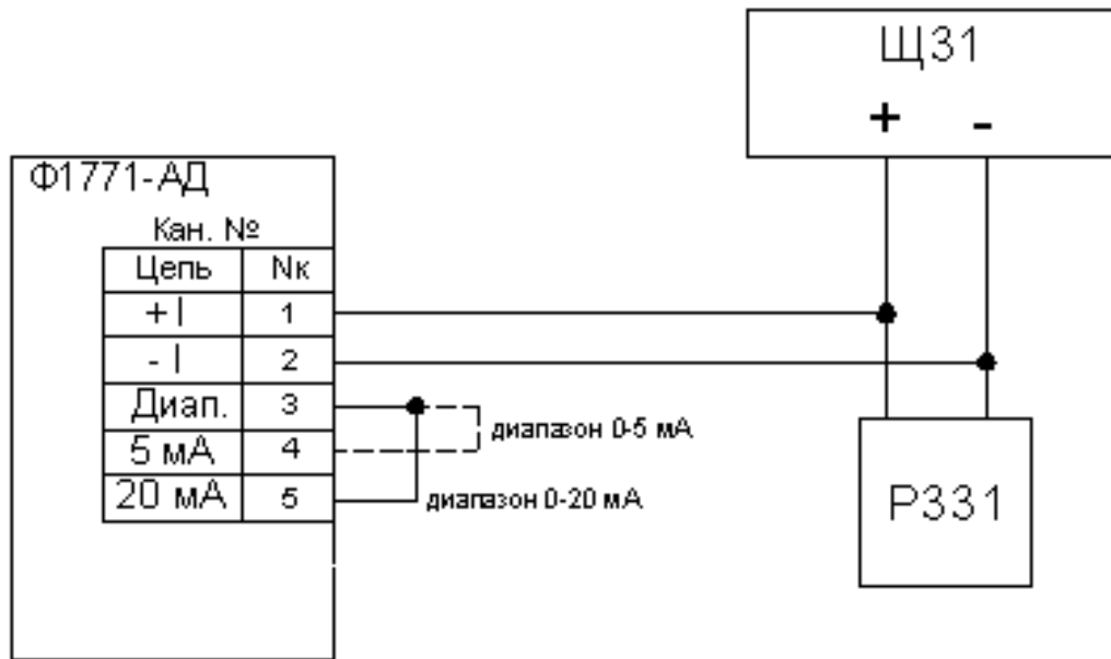
Рисунок 66 – Сема подключения выходного канала.
