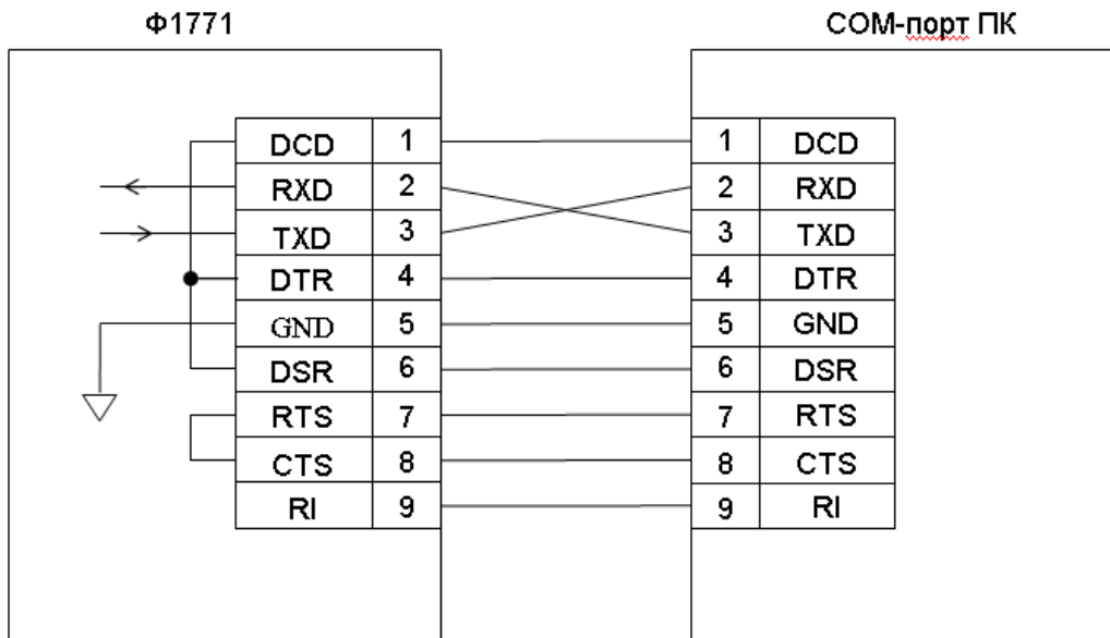
Рисунок 59 – Схема подключения к ПК по интерфейсу RS232
