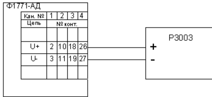
Рисунок 61 – Схема подключения входных каналов для U в диапазонах до \pm 1000 мВ и сигналов ТП
